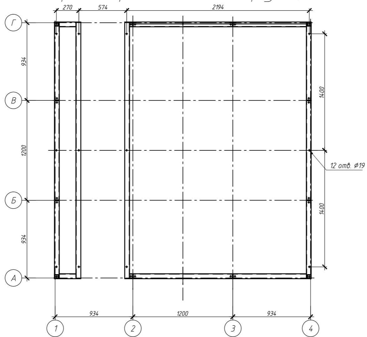
Опорная рама. Конструкция.
